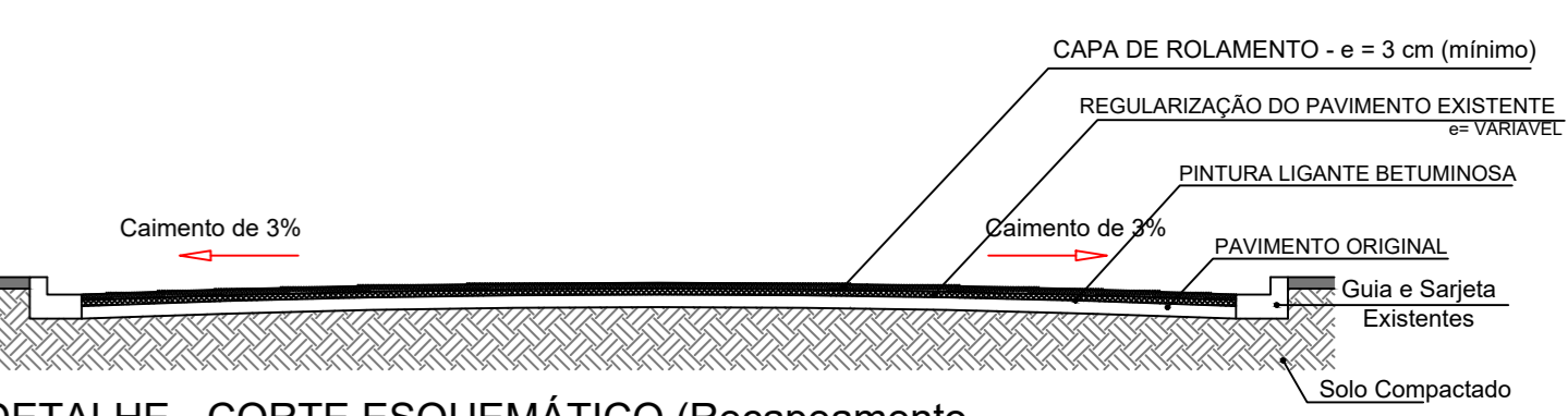
DETALHE - CORTE ESQUEMÁTICO (Recapeamento Asfáltico) s/ escala
