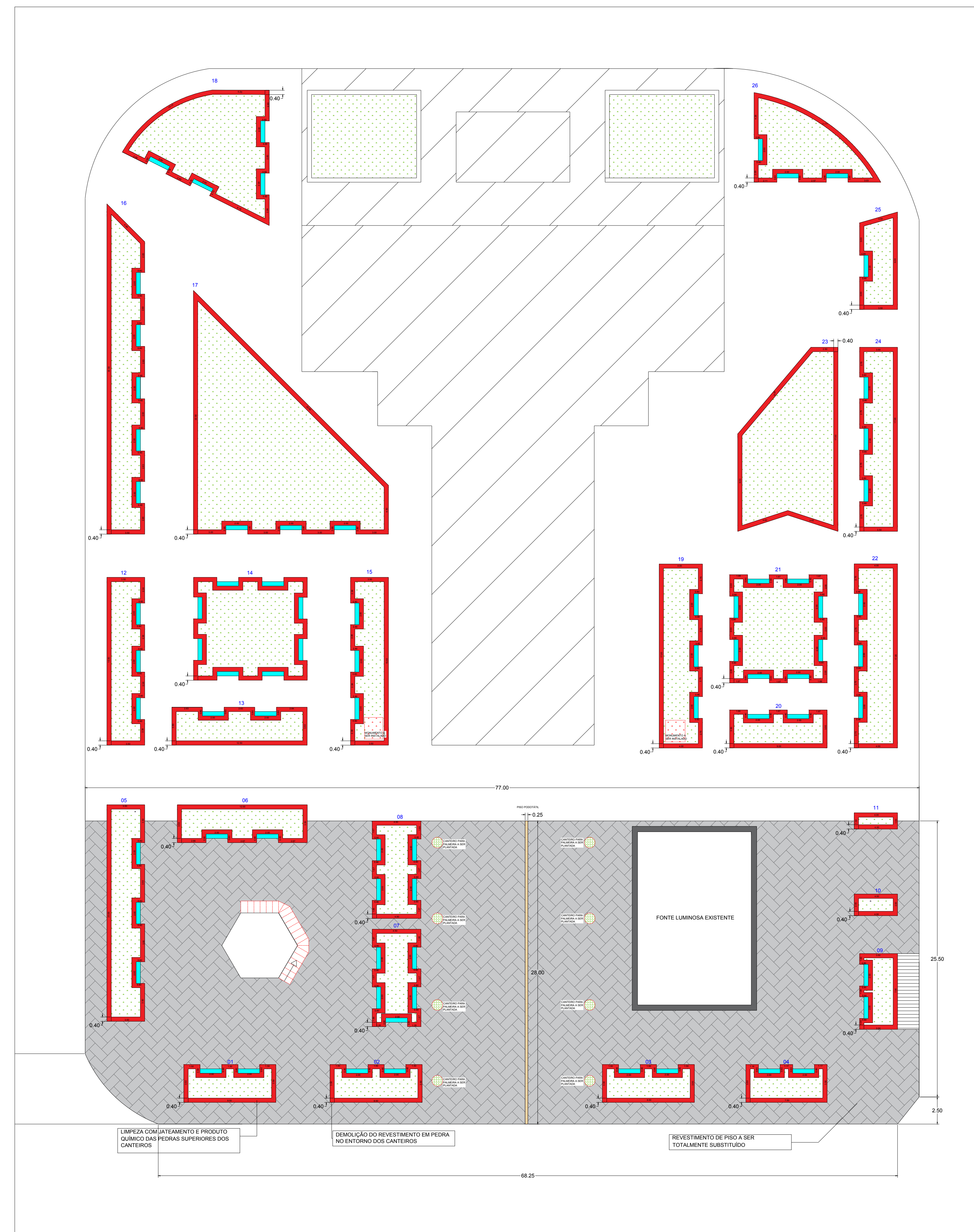
DETALHES DAS ÁREAS A CONSTRUIR escala 1:200
