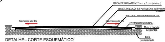
DETALHE - CORTE ESQUEMÁTICO (Recapeamento Asfáltico) s/ escala
