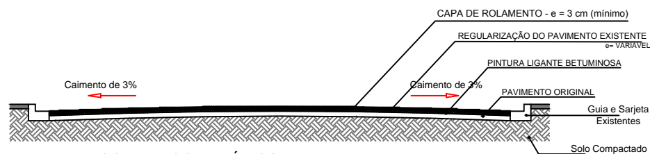
DETALHE - CORTE ESQUEMÁTICO (Recapeamento Asfáltico) s/ escala
