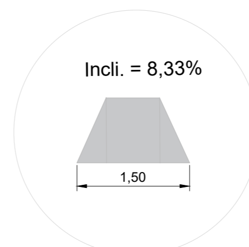
Detalhe Rampa de Acessibilidade Sem Escala
