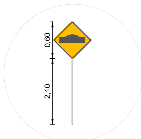
Detalhe placa de sinalização Sem Escala
