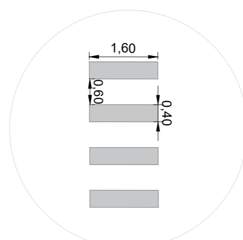
Detalhe faixa de pedestre Sem Escala
