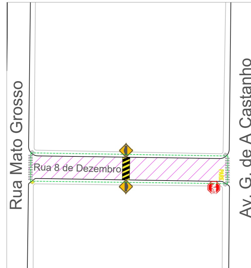
RUA 08 DE DEZEMBRO (TRECHO 02) Esc.: 1:1000
