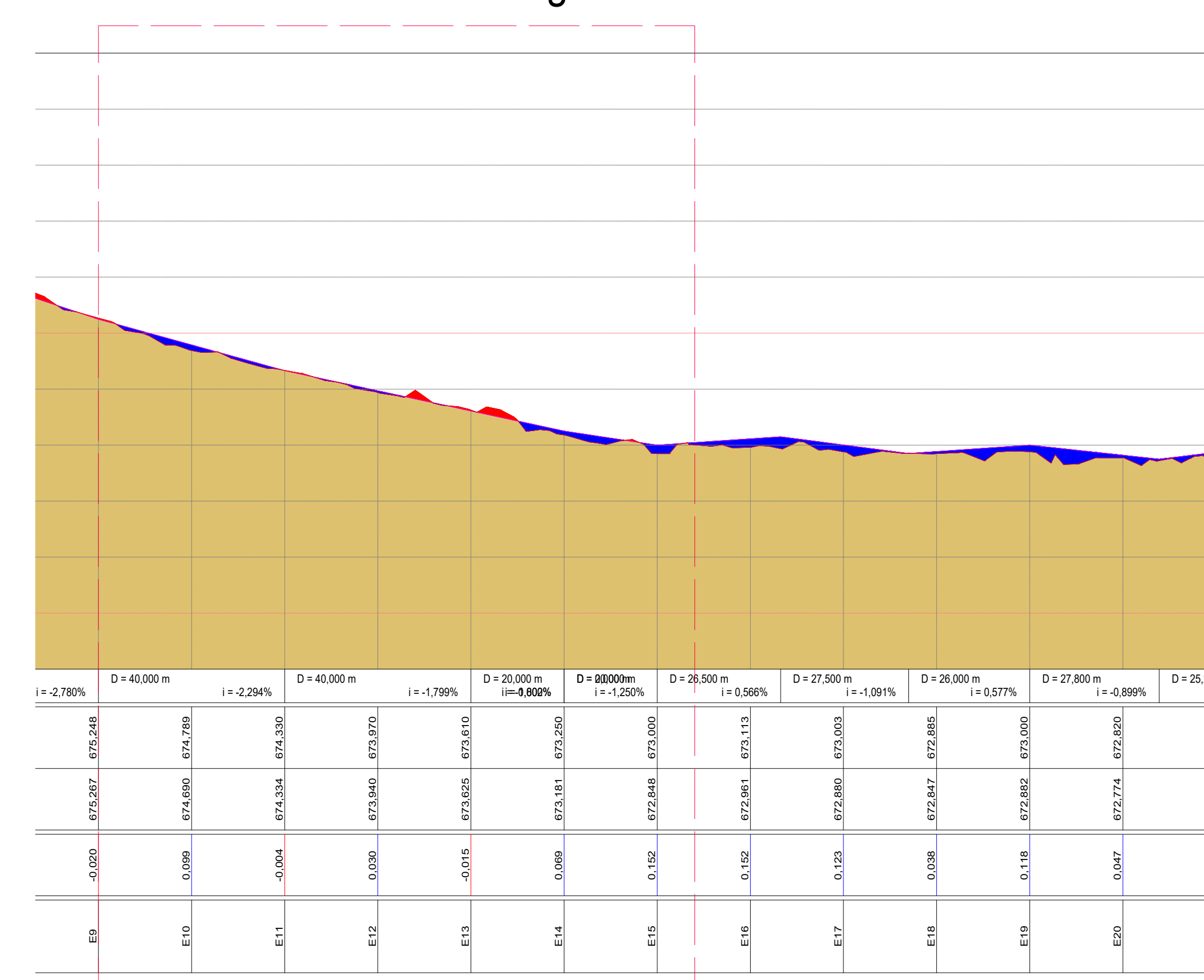
Perfil longitudinal da Rua Irineu Paschoal Trecho a ser pavimentado na Fase 2 Esc.: 1:1000
