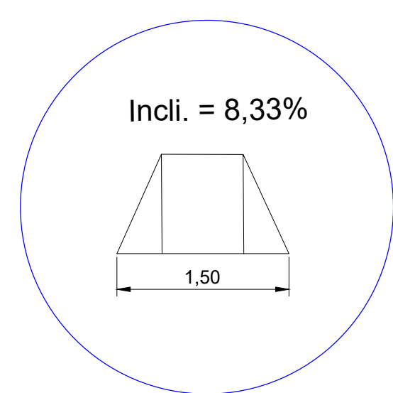
Detalhe Rampa de Acessibilidade Sem Escala
