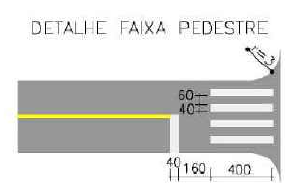
Detalhe: Faixa de Pedestre Sem escala
