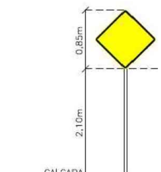
Detalhe: Placa de Sinalização Sem escala
