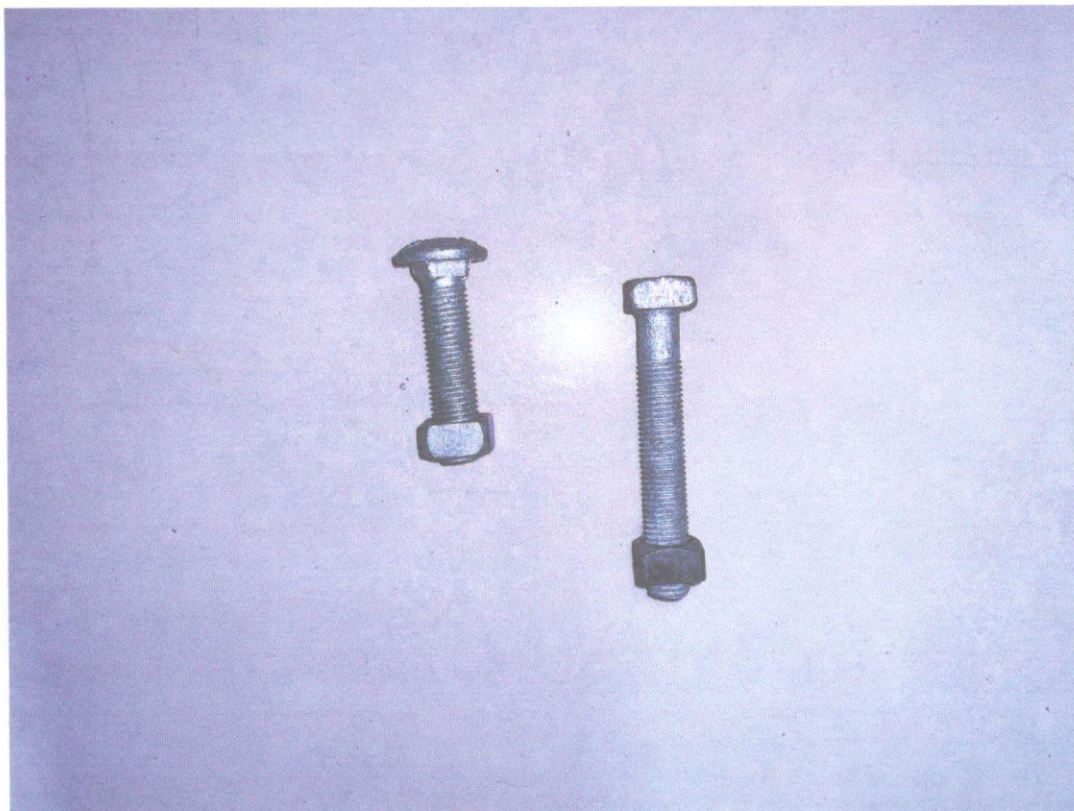
Parafuso Sextavado Rosca Inteira M16-2,00MA-70 e Porca Sextavada M16-2,00Ma-Chave 24
